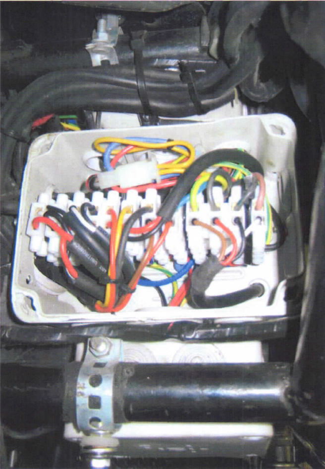
Kabeldose Mitte mit grünen Klemmen
